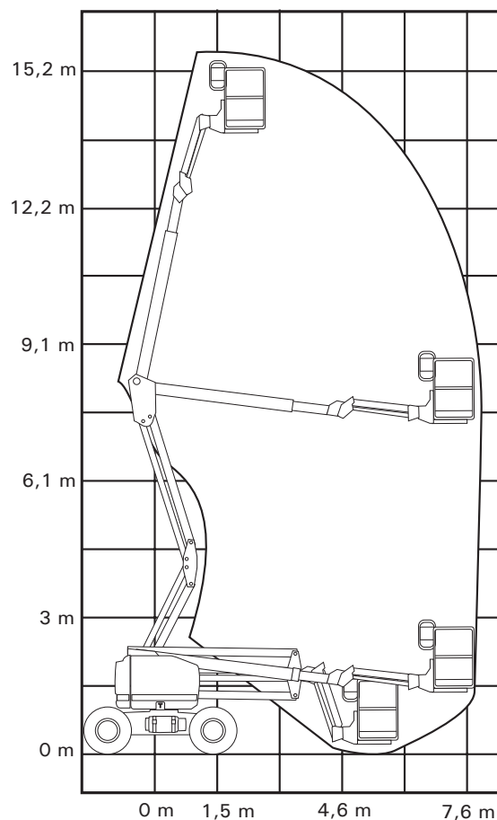
Envelope de trabalho - modelos com jib
